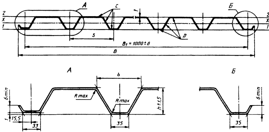
Рисунок 9 - Профилированный лист типа С высотой 21 и 44 мм
