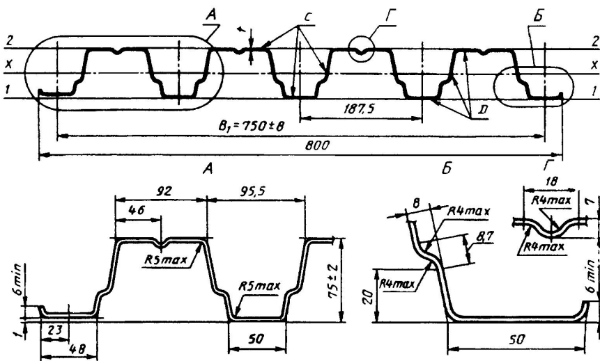
Рисунок 2 - Профилированный лист типа Н высотой 75 мм
