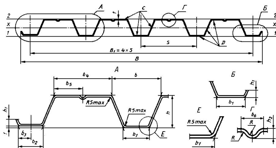
Рисунок 1 - Профилированный лист типа Н высотой 57 и 60 мм
