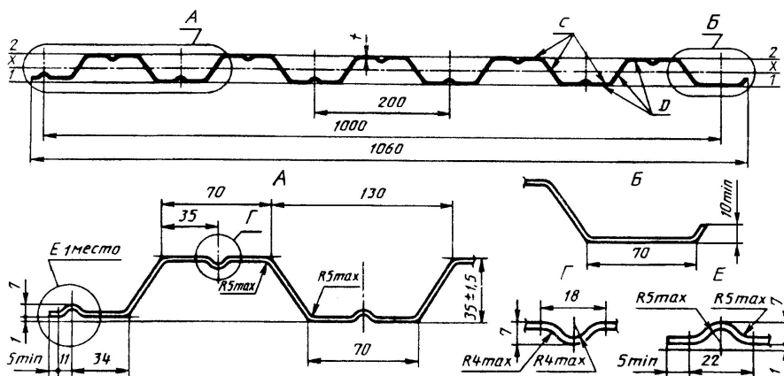
Рисунок 5 - Профилированный лист типа НС высотой 35 мм
